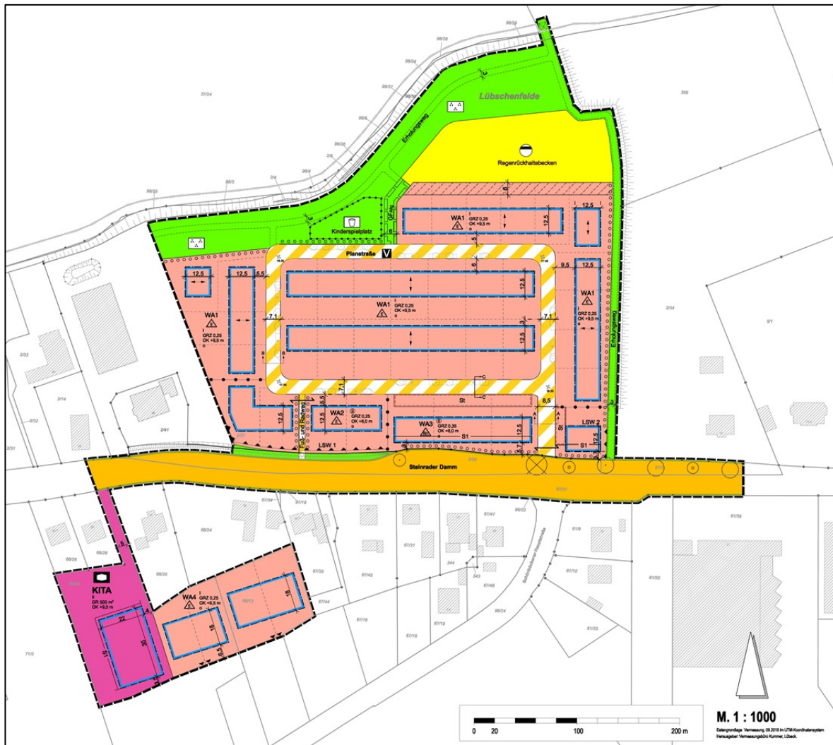
Abbildung 3: B-Plan-Entwurf (Stand: 08.03.2021)
